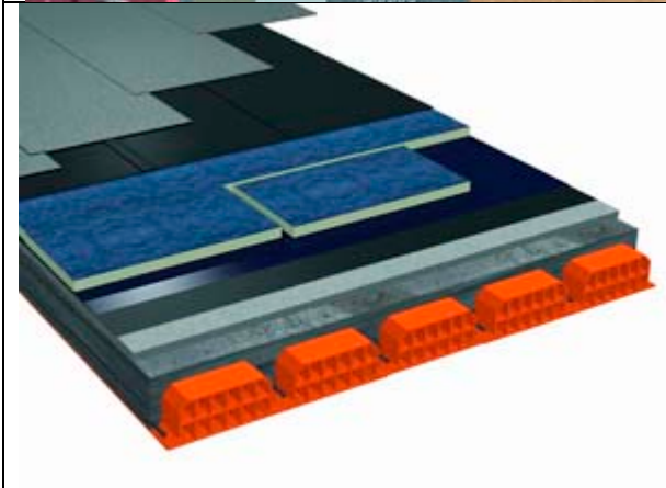
Stratigrafia copertura
